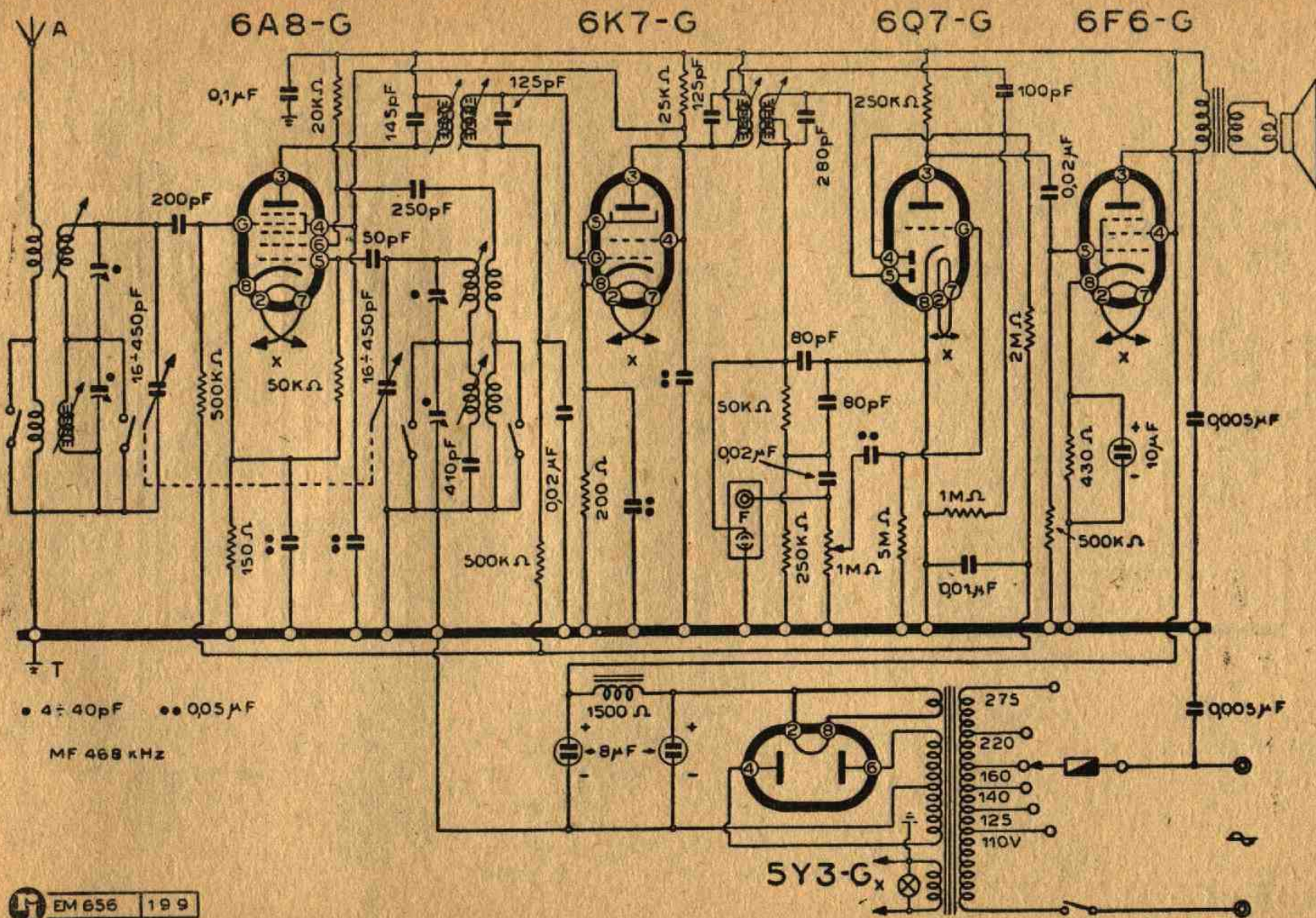
Lo schema elettrico del C.G.E. mod. 365
